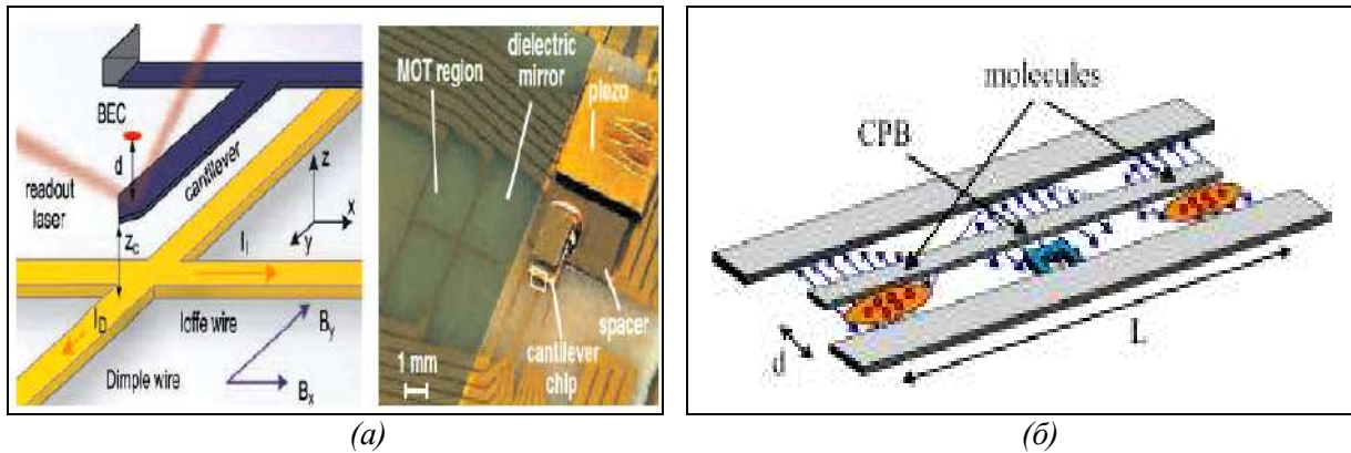
Рис. 5. Конденсат Бозе-Эйнштейна на атомном чипе, встроенном в консоль [1]; Движение консоли воспроизводит потенциал атомов, которые приводят в связанное движение в консоле (слева – вид устройства; вибрации консоли с атомами регистрируются с помощью луча лазера; слева – фотография устройства) (а); и Блок формирования кубита на паре Купера и ансамбле поляризованных молекул (связанных состояний в микроволновой полосе фотонов. Строгая связанность состояний достигается на квазиодномерной структуре длиной порядка см и шириной порядка мкм) [16]) (б)
