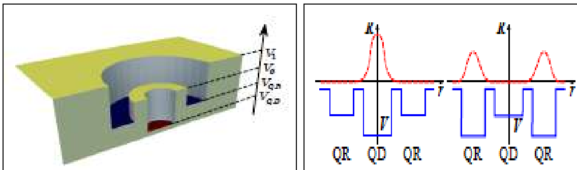
Рис. 6. Разрез квантовой точки с указанием потенциальных барьеров тунnelирования (а); и виды основных и возбужденных состояний волновых функций при различных соотношениях высоты потенциальных барьеров (б)
