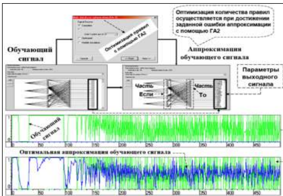
Рис. 3. Пример оптимизации количества продукционных правил при аппроксимации сигнала обучения с заданной ошибкой аппроксимации
