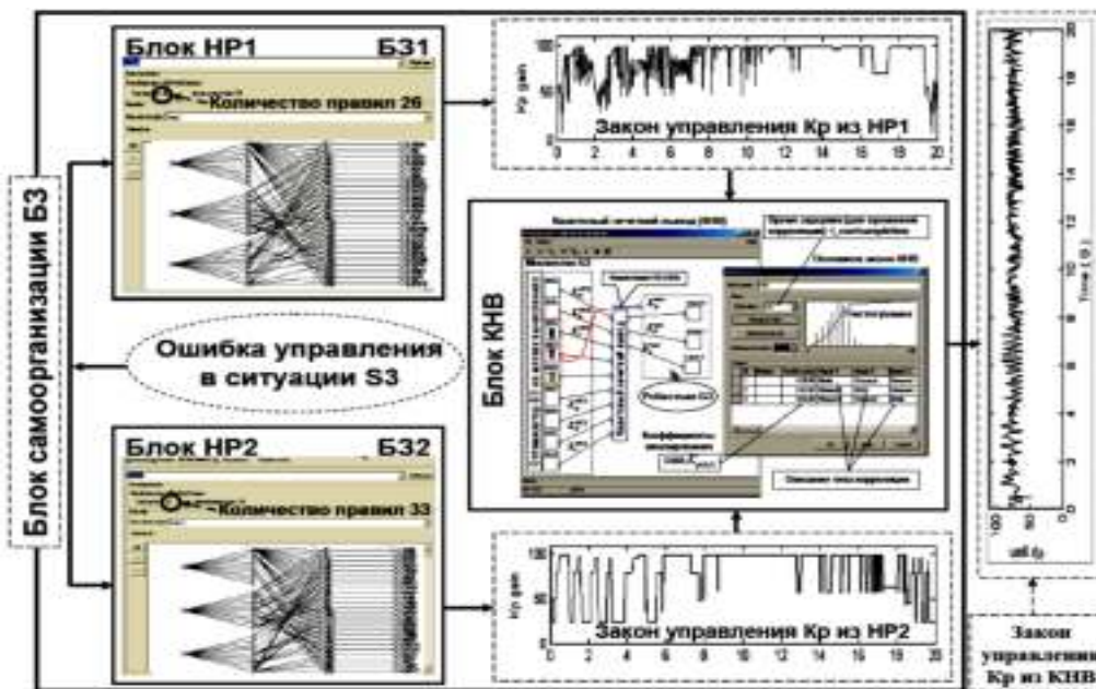
Рис. 18. Пример работы блока самоорганизации БЗ на основе КНВ
