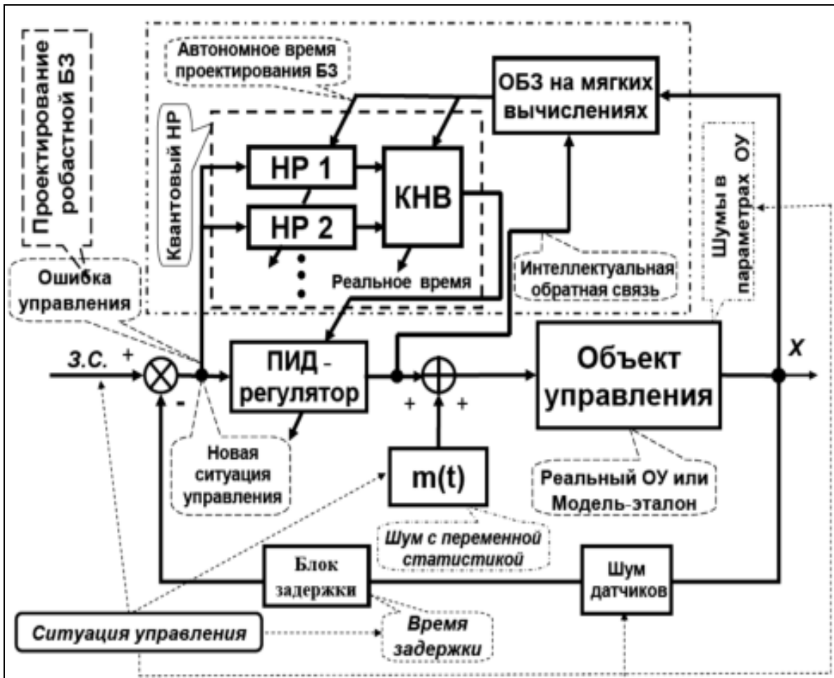
Рис. 13. Структура ИСУ с ОБЗ на мягких вычислениях и квантовых вычислениях
