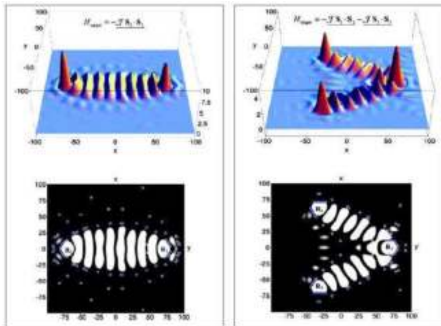
Рис. 11. Пример влияние типа квантовой корреляции между спинами на вид наноструктуры квантового «коралла»
