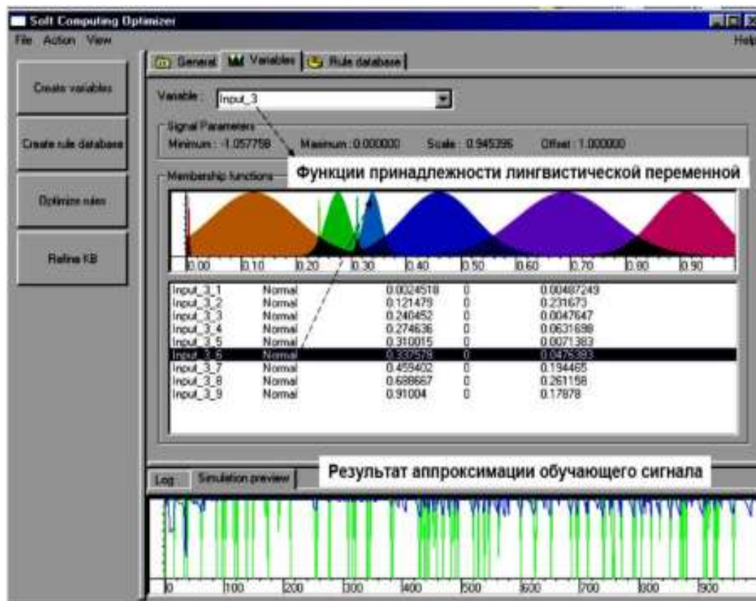
Рис. 16. Пример оптимального вида функций принадлежности для третьей выходной переменной k_I (коэффициент усиления интегральной ошибки)
