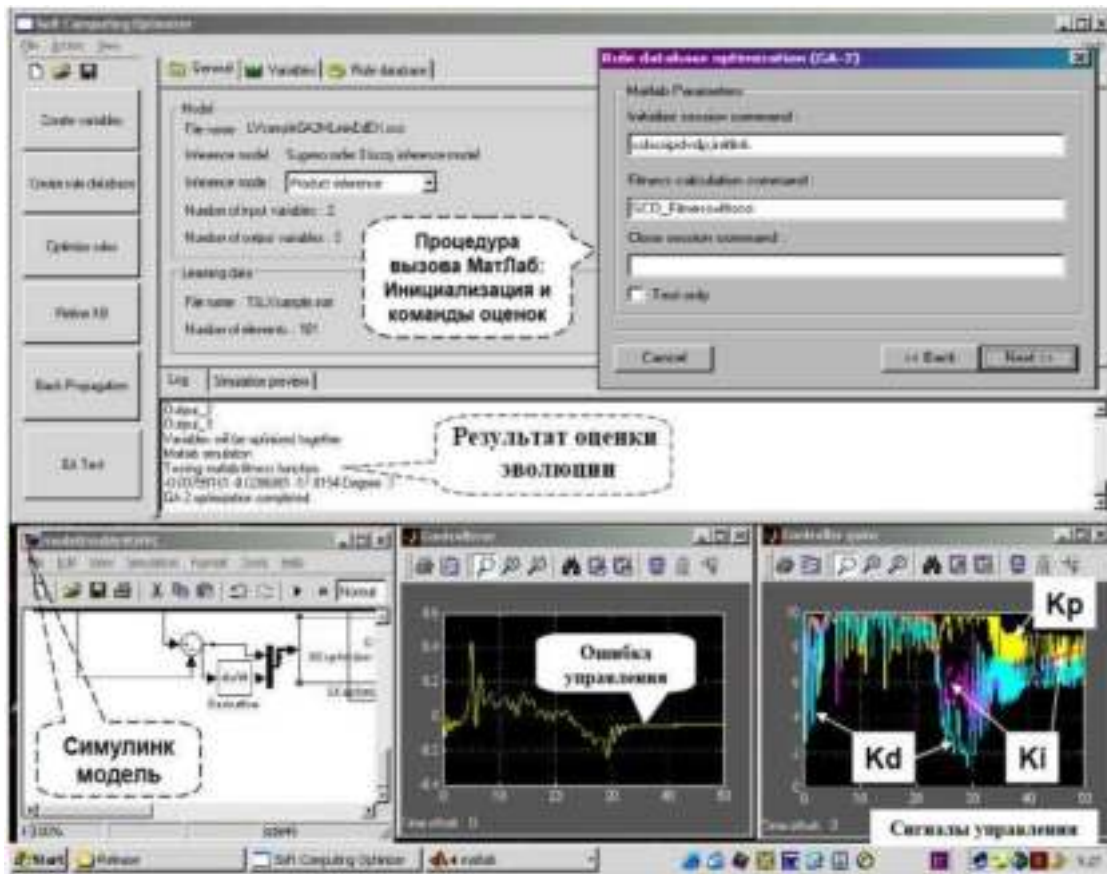
Рис. 4. Пример проектирования законов управления коэффициентами усиления нечеткого ПИД-регулятора с заданной ошибкой аппроксимации ОС
