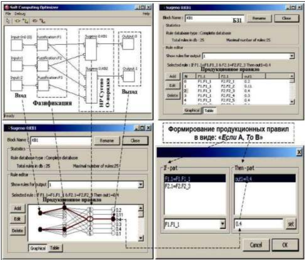
Рис. 14. Структура моделирования НР и программная поддержка проектирования БЗ
